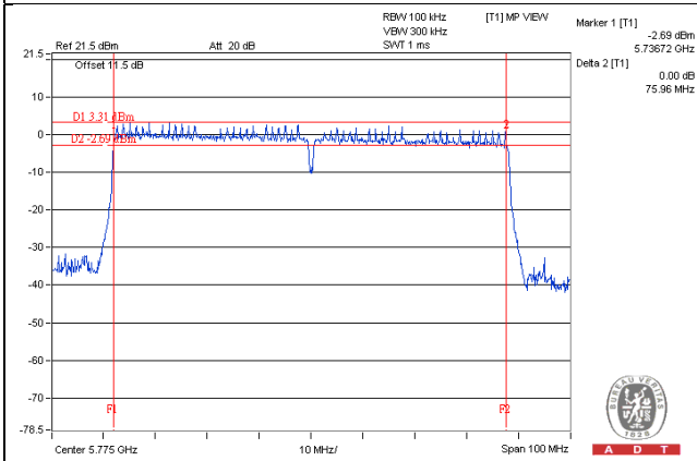
802.11ac (80MHz+80MHz)
