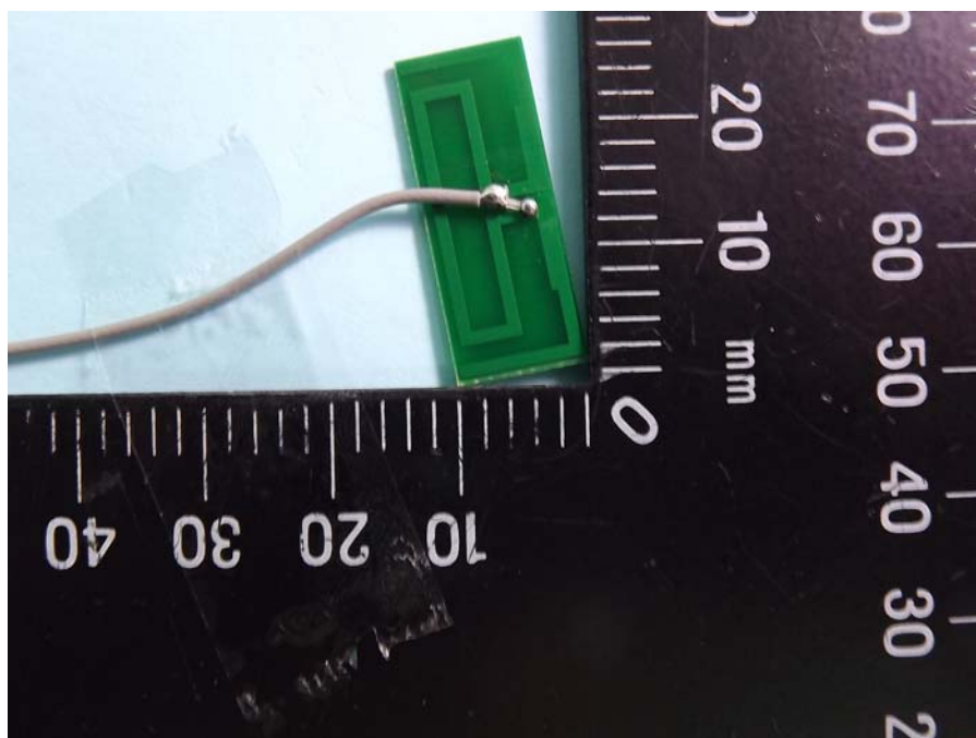
5GHz WLAN Module
