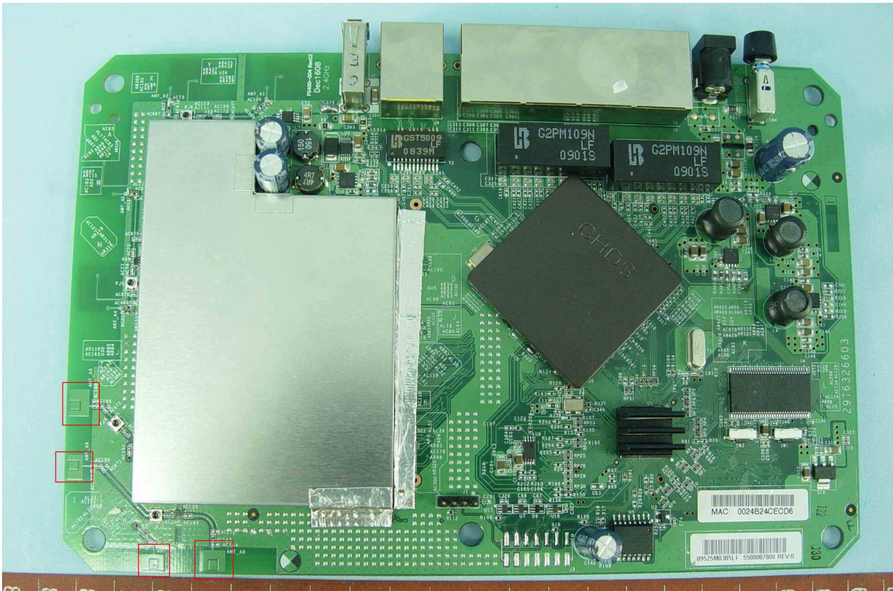
2.4GHz antenna
