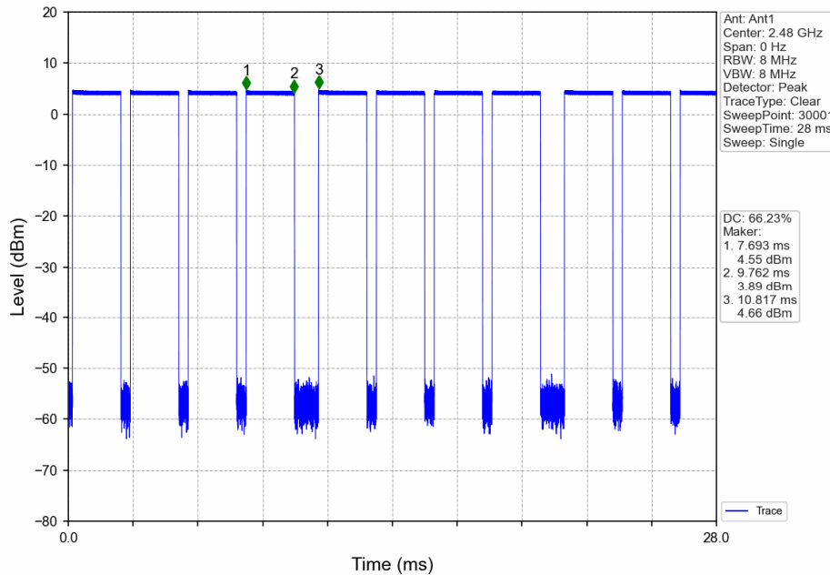
1M_HCH_2480MHz_DataRate=_Ant1_NTNV
