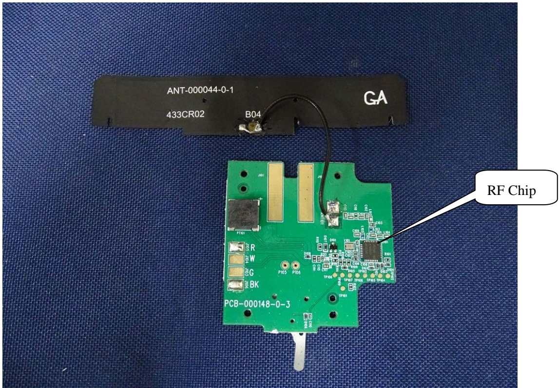
(10) EUT Photo
