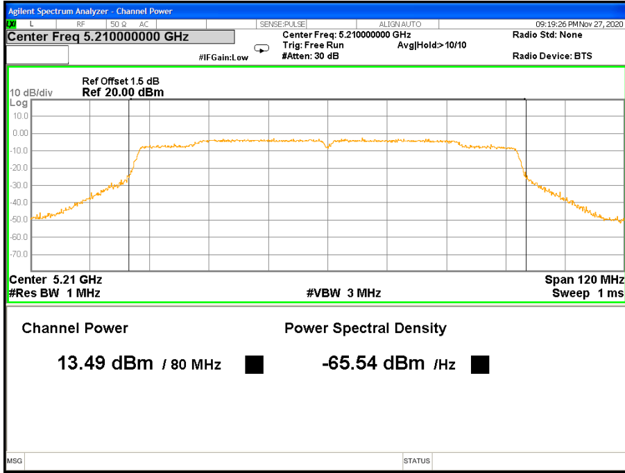
5210MHz_AV_Ant A
