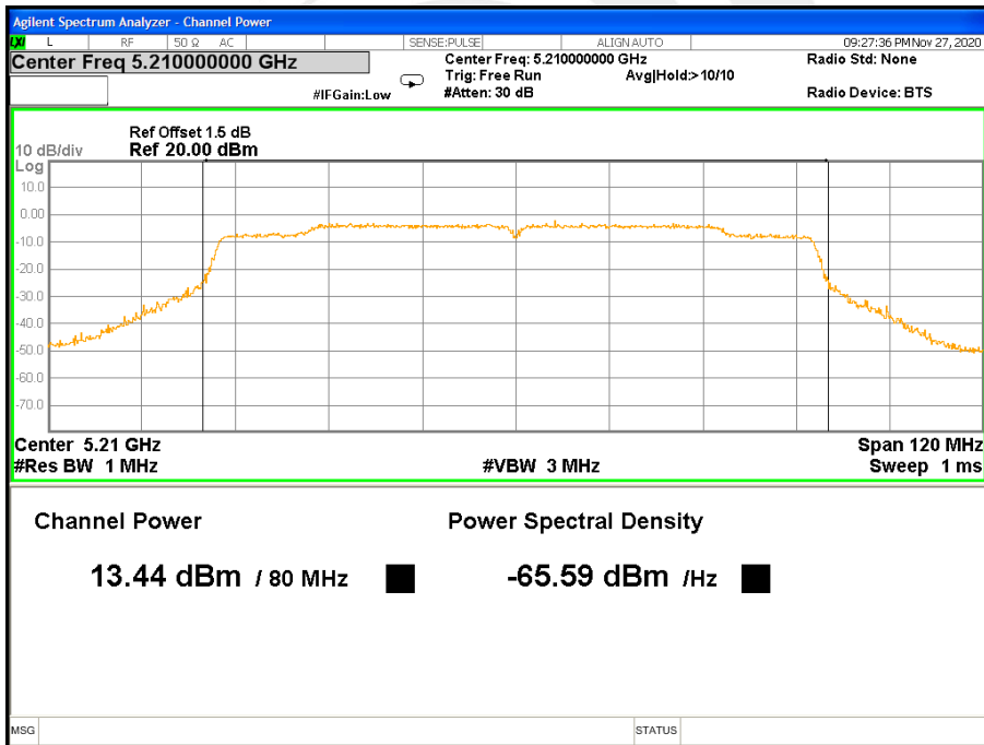
5210MHz_AV_Ant B
