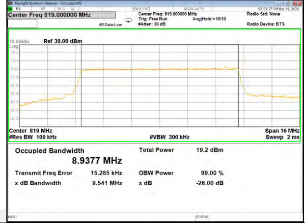
B26_Q16_10M_Mid_26BW-99%
