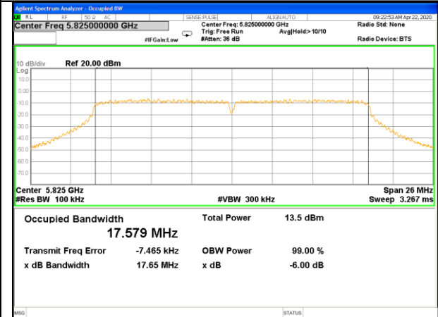
W58_11ac20_Higher_6BW
