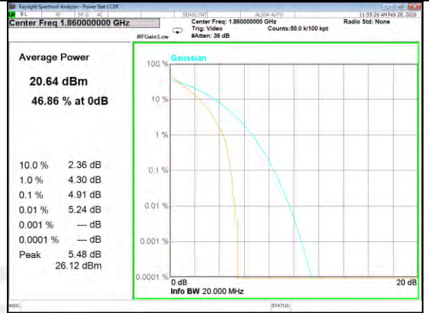
B2_100_Q16_Lower_
