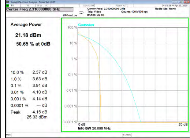
B30_1_Q16_Middle_
