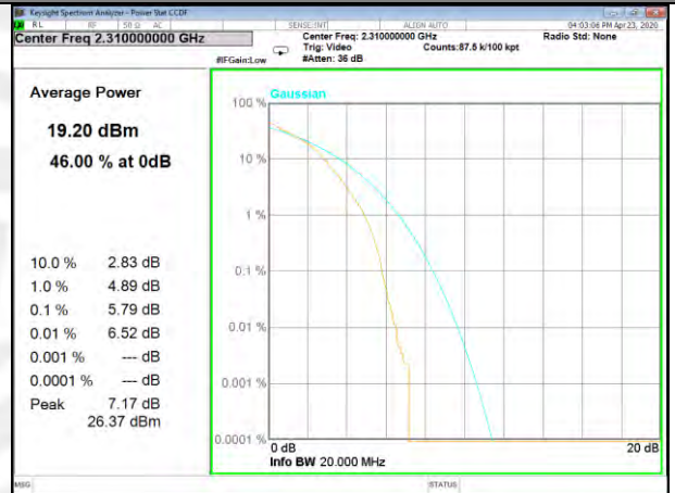
B30_50_Q16_Middle_
