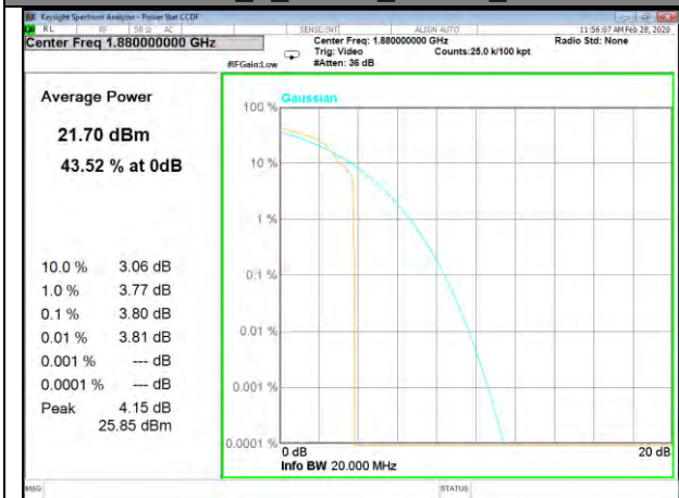
B2_1_QPSK_Middle_
