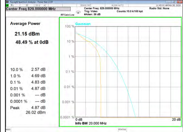
B5_1_Q16_Lower_
