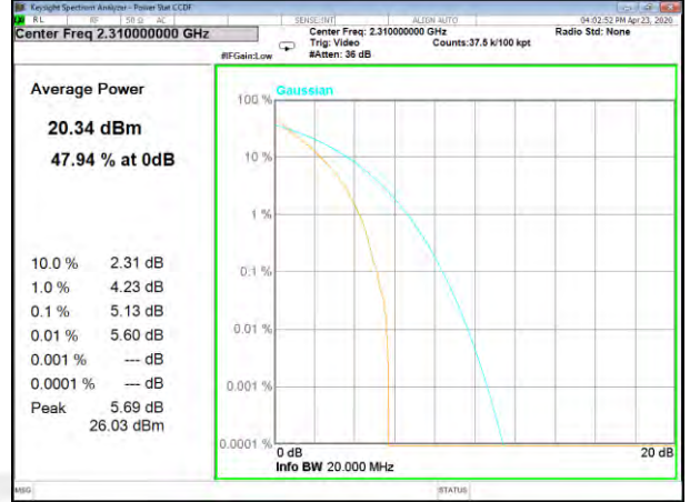
B30_50_Q16_Middle_
