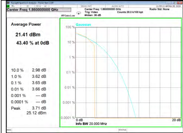
B2_1_Q16_Lower_
