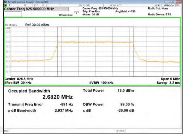
B26_Q16_3M_Mid_26BW-99%
