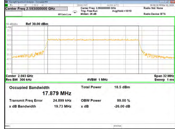
B41_Q16_20M_Mid_26BW-99%
