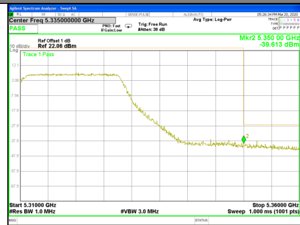
W53_11ac40_Higher_Band edge
