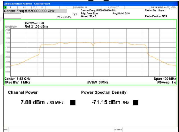
5530MHz AV Ant B
