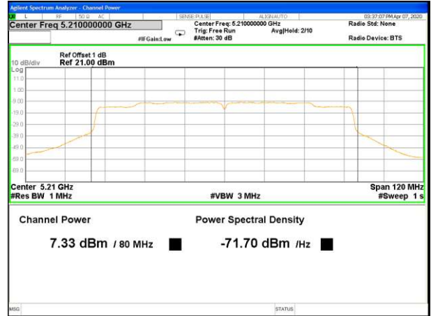
5210MHz AV Ant B
