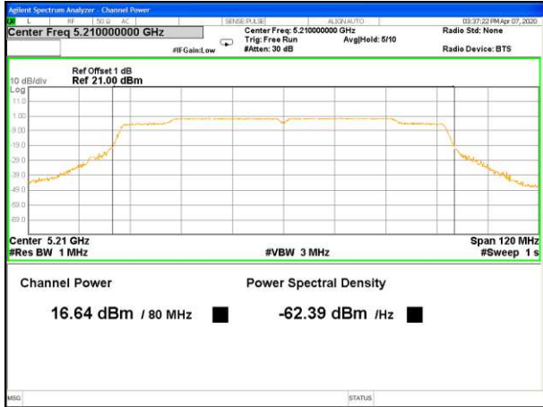
5210MHz PK Ant B
