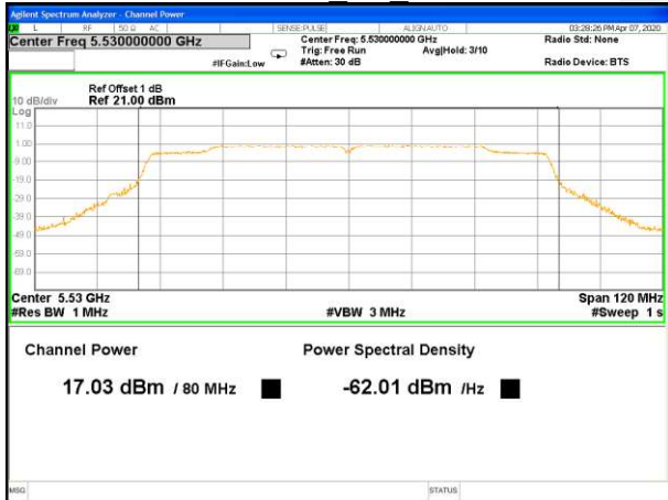
5530MHz PK Ant B
