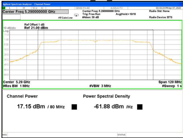
5290MHz PK Ant A
