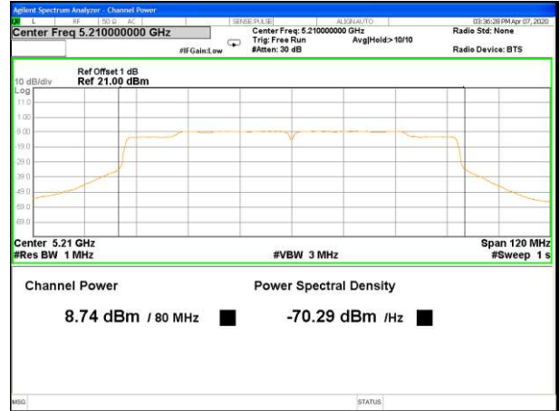
5210MHz AV Ant A
