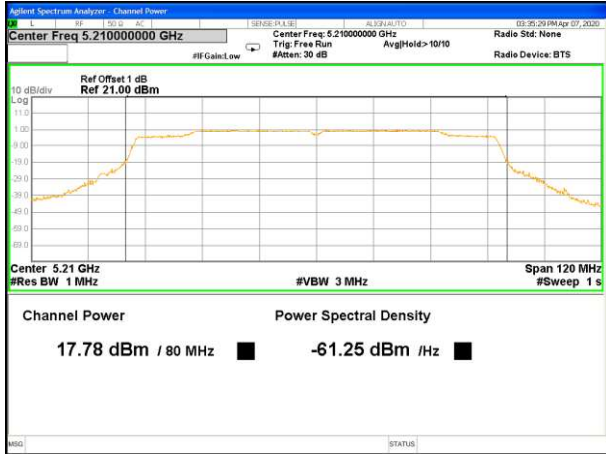
5210MHz PK Ant A
