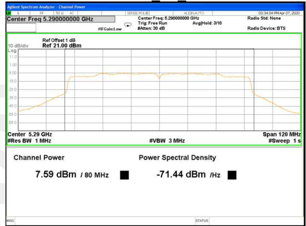
5290MHz AV Ant A
