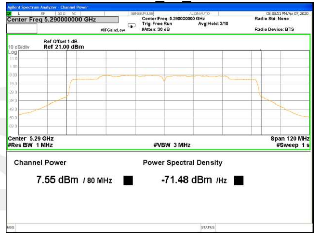
5290MHz AV Ant B
