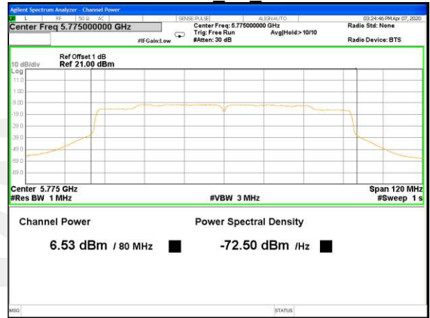
5775MHz AV Ant A
