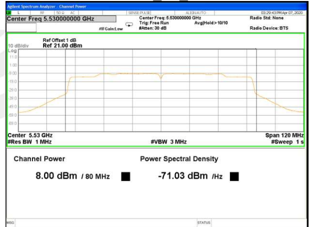
5530MHz_AV_Ant A
