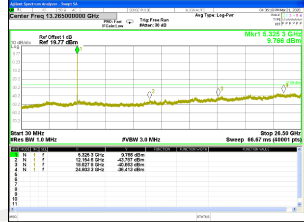
W53_11n20_Higher_Band edge
