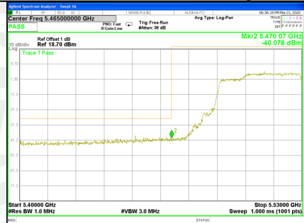
W56_11ac80_Lower_Band edge
