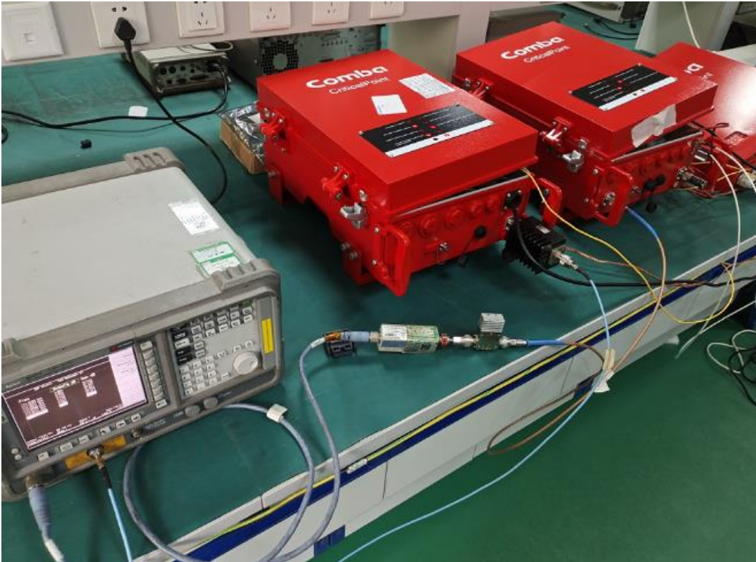
Test scenario-3
