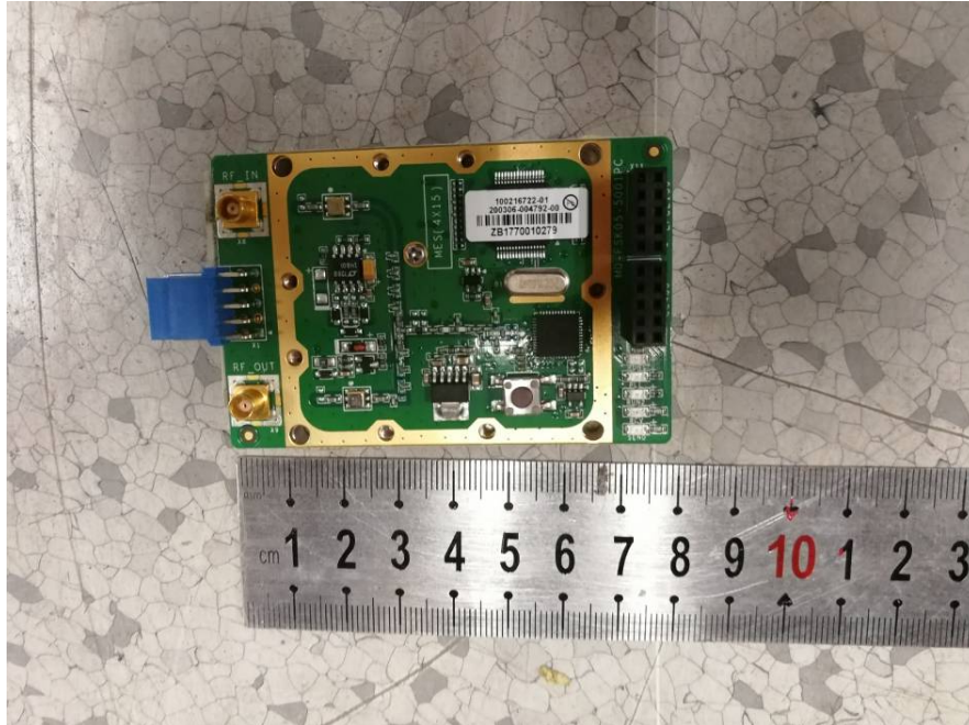
EUT – FSK Module Top View
