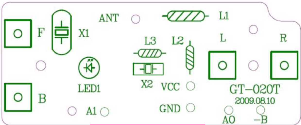
TOP SILKGREEN
