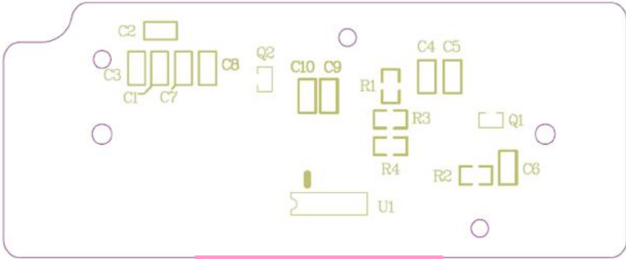
BOTTOM SILKGREEN
