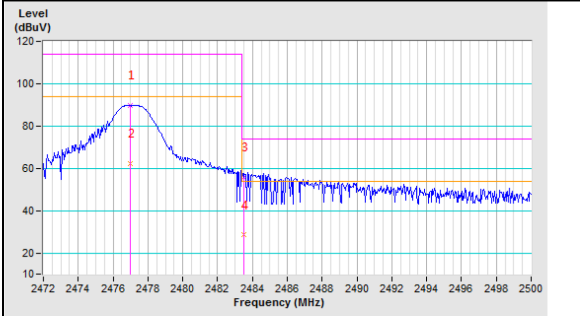
2477MHz Vertical
