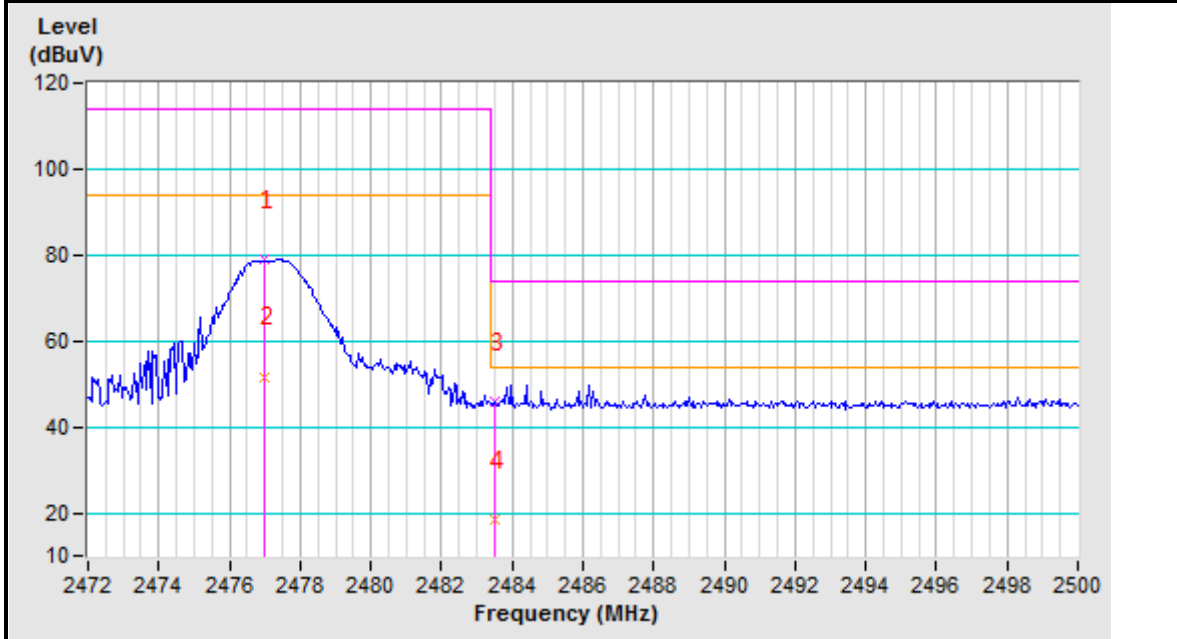
2477MHz Vertical
