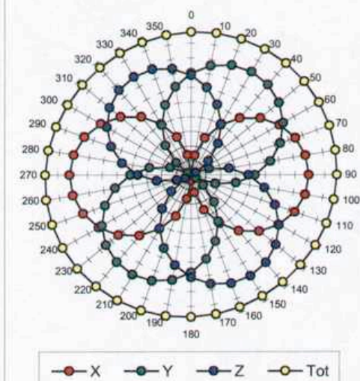
f = 600 MHz, TEM ifi110EXX
