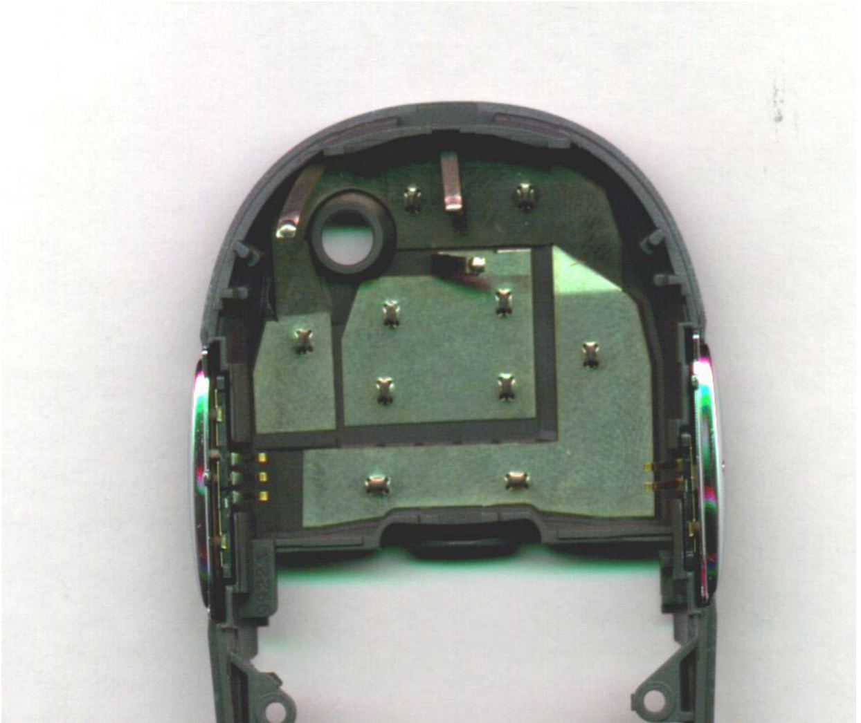
GSM Antenna
