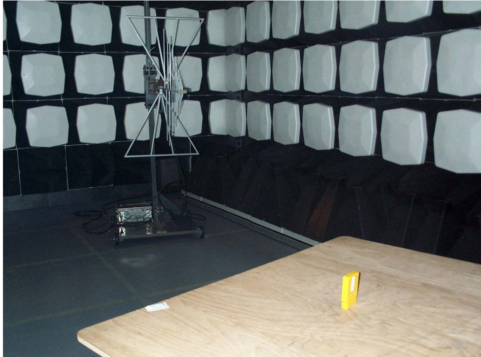
Bild 2. El. Funkstörfeldstärke [emission, radiated disturbance]
