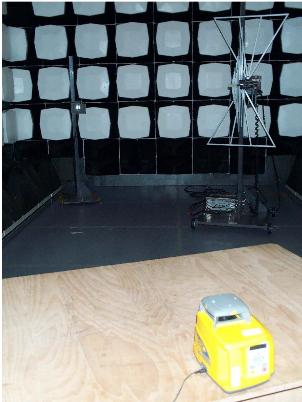
Bild 3. El. Funkstörfeldstärke [emission, radiated disturbance]
