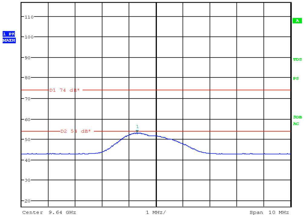
Picture 50: spurious emission, Channel low - AV
