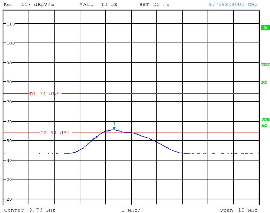
Picture 56: spurious emission, Channel mid - AV
