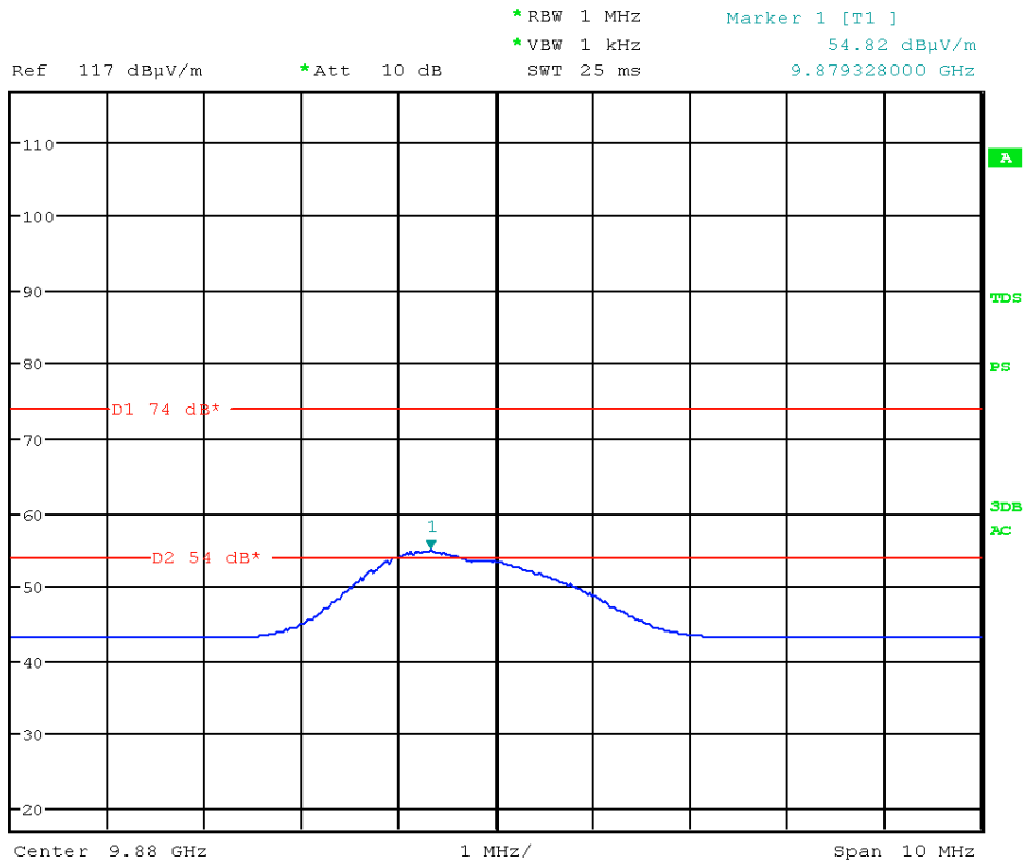
Picture 62: spurious emission, Channel mid - AV
