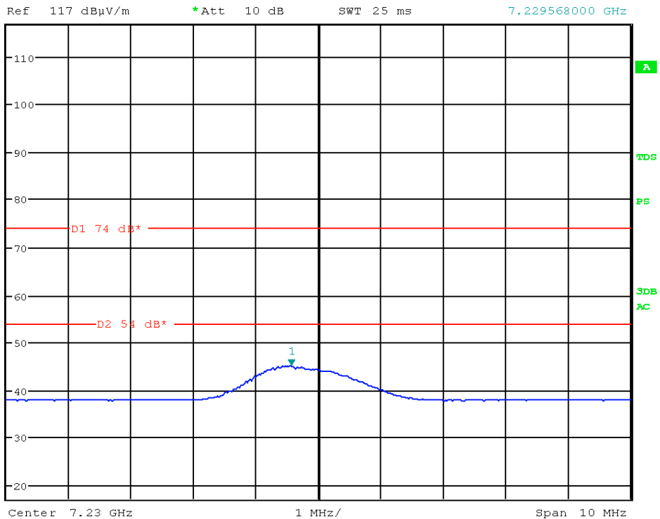
Picture 48: spurious emission, Channel low - AV
