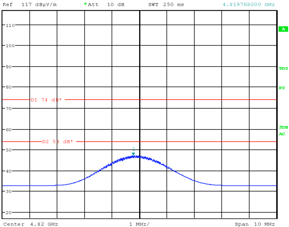
Picture 46: spurious emission, Channel low – AV
