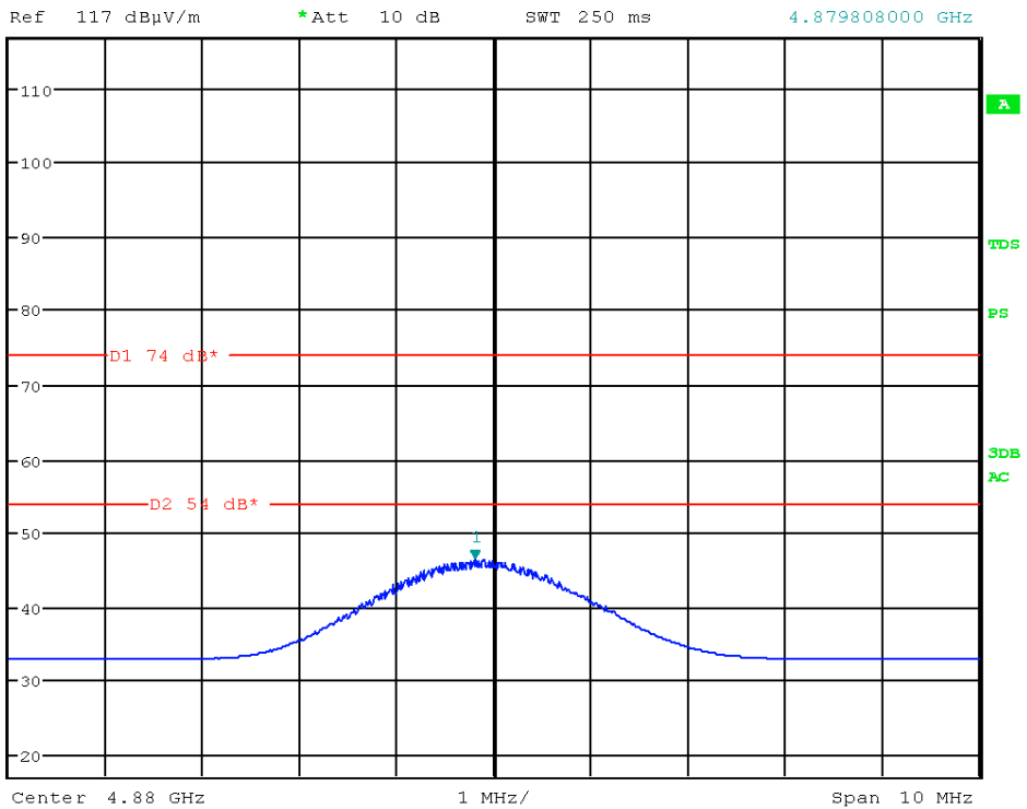
Picture 54: spurious emission, Channel mid – AV
