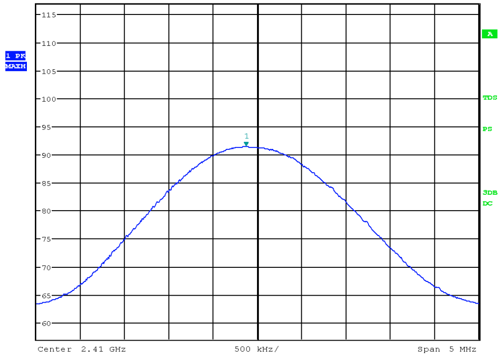
Picture 44: spurious emission, Channel low - AV
