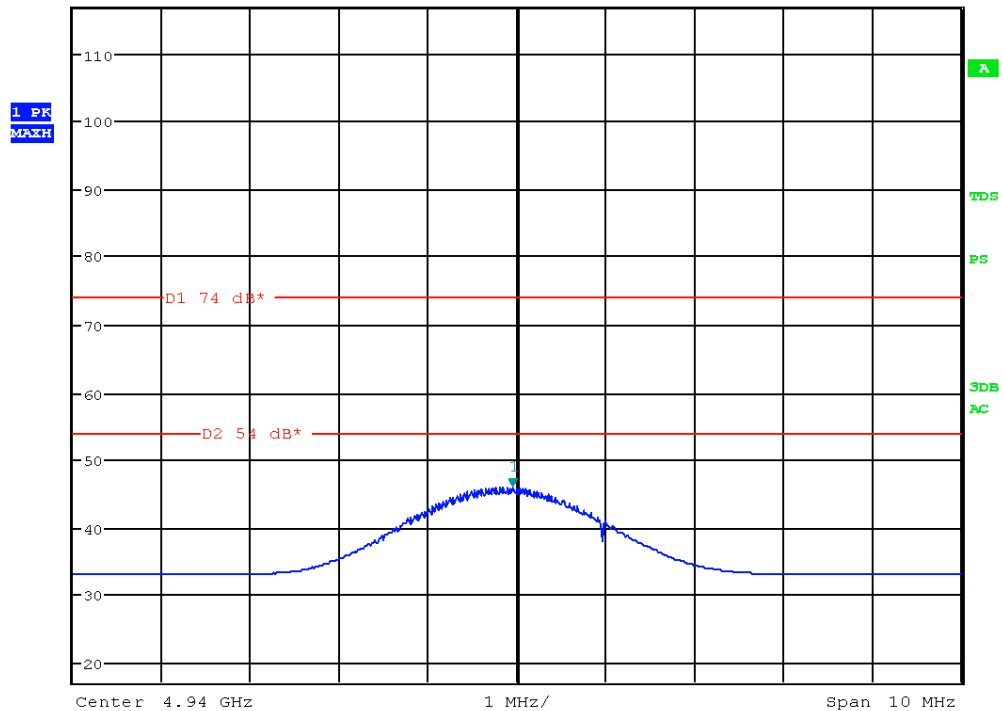
Picture 60: spurious emission, Channel high - AV
