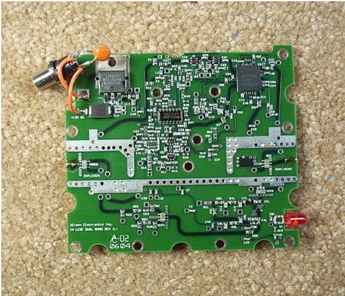
PCB Top
