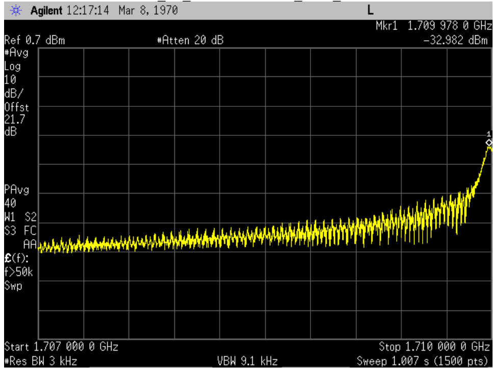
OOBE_UL_1710 - 1755 MHz_GSM_Lower
