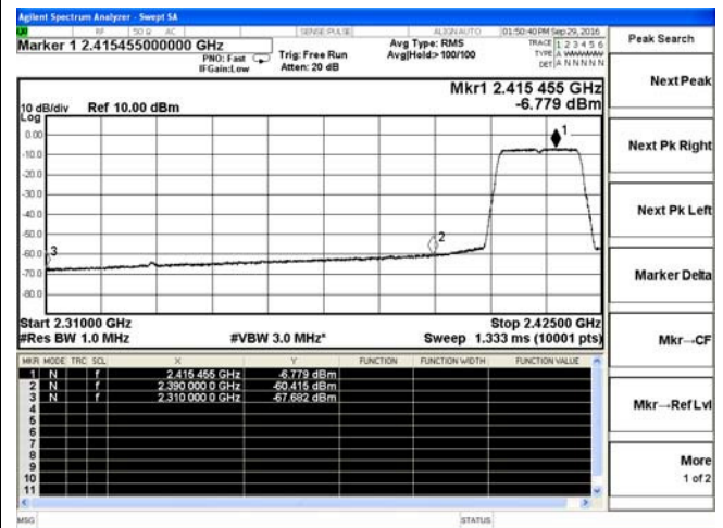
802.11g-Low channel(Average)
