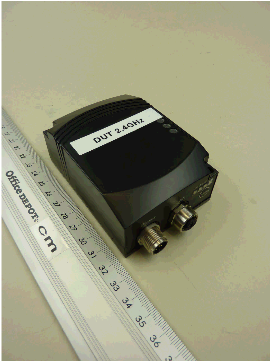
101042_a.jpg cB-RWE231, 3-D-view 1
