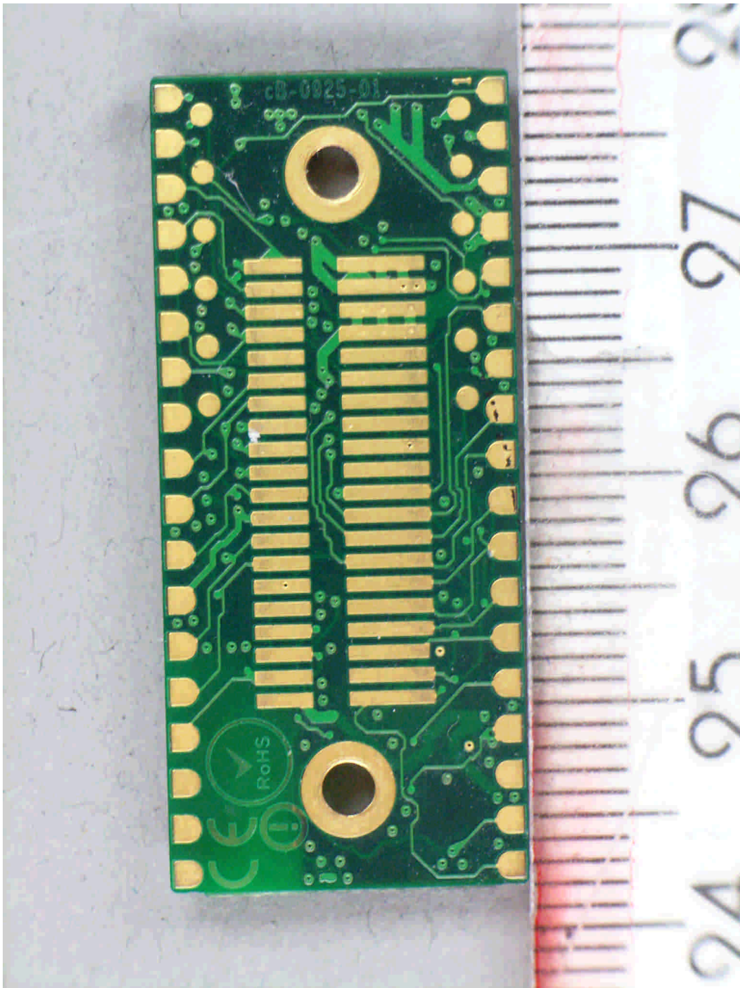
103572_g.jpg cB-0925-01-1-0x, bottom view
