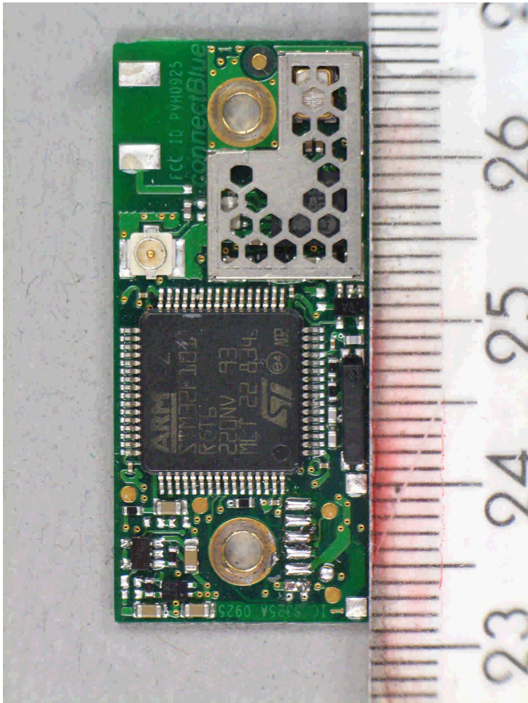
103572_d.jpg cb-0925-01-1-02, top view
