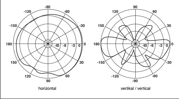
Richtcharakteristik / Radiation pattern / Diagramme de rayonnement / Característica direccional
