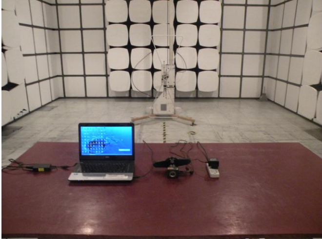
Below 1G
