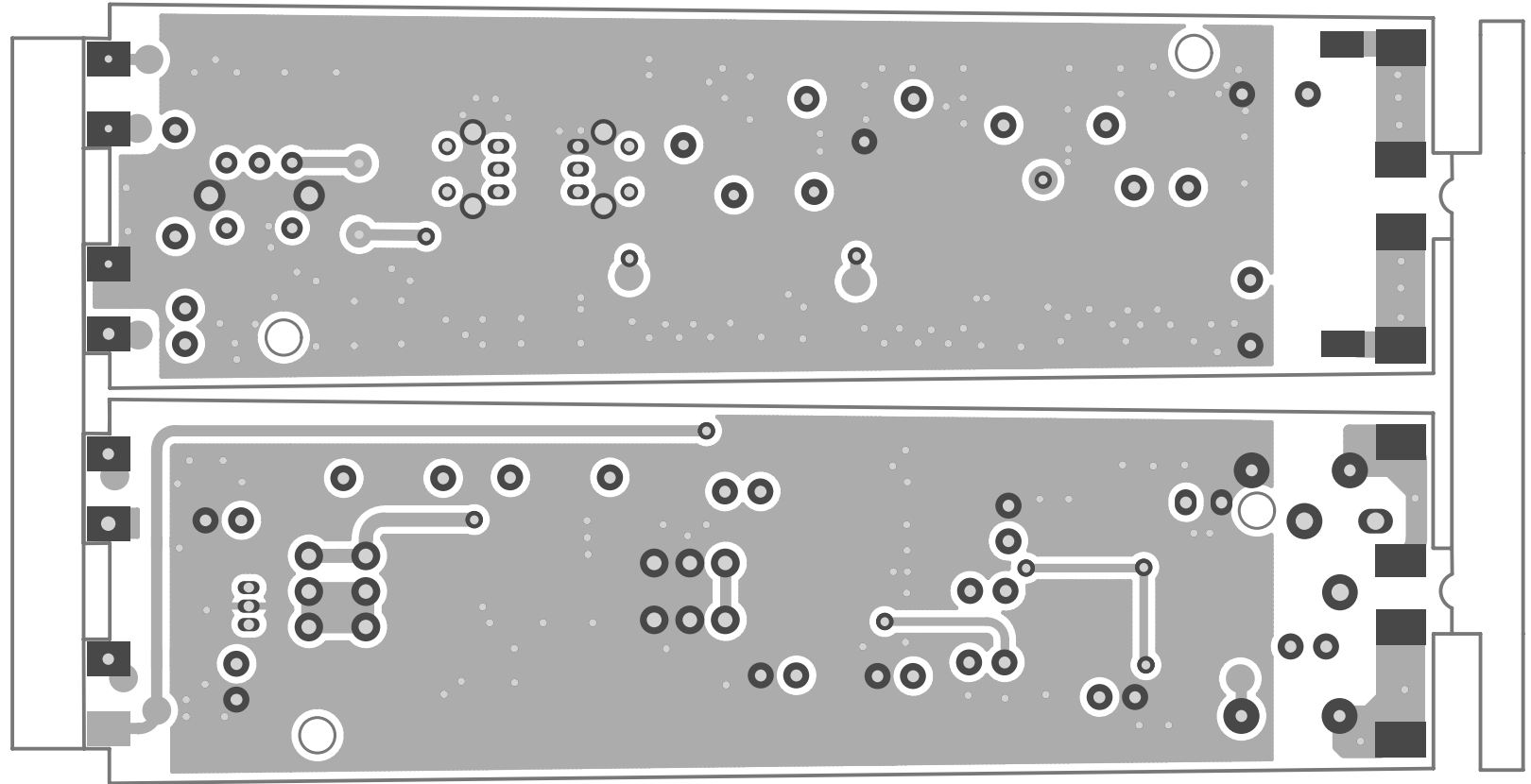
HT-U20 Transmitter Bottom Layer
