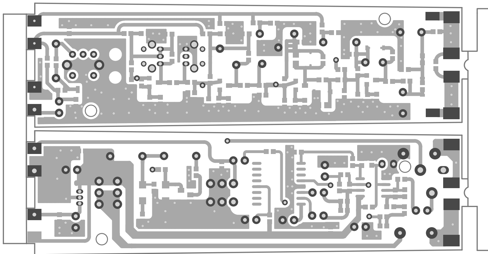
HT-U20 Transmitter Top Layer
