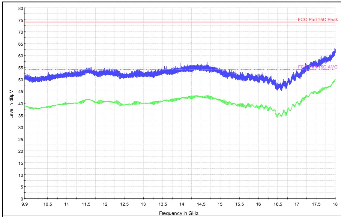
Frequency range:9.9GHz-18GHz
