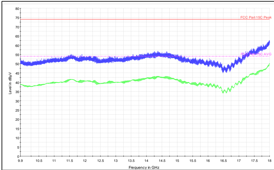
Frequency range:9.9GHz-18GHz
