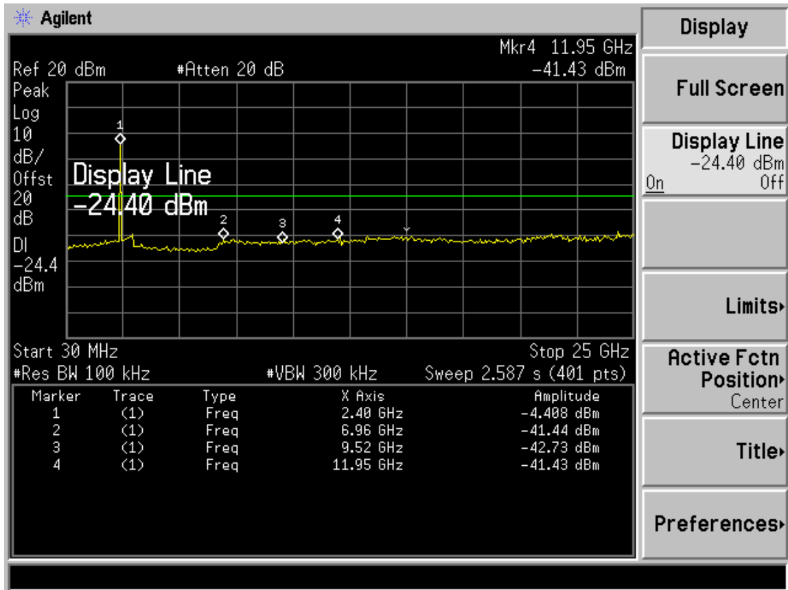
802.11b CH6
