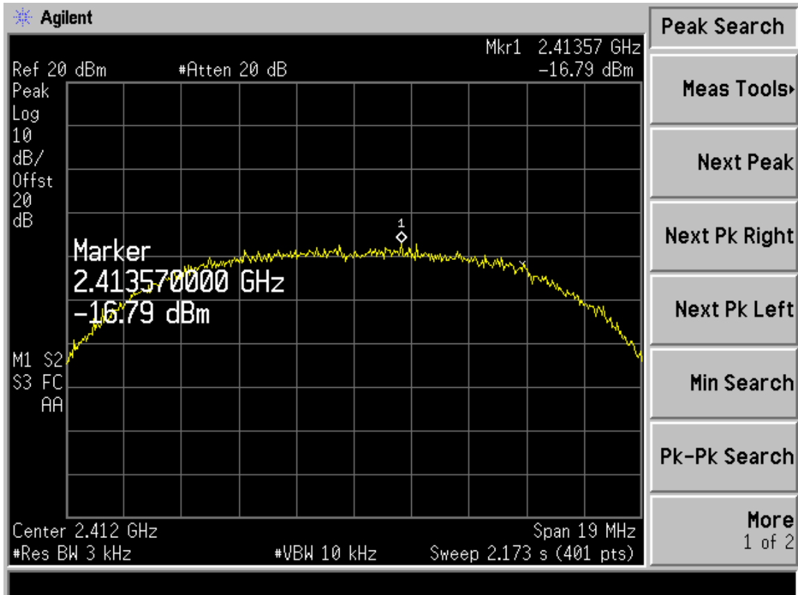
802.11b CH6
