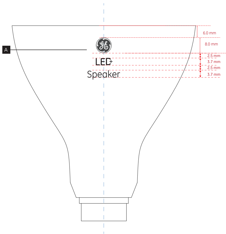
BR30(TCO)LED灯2700K版本(正面)
