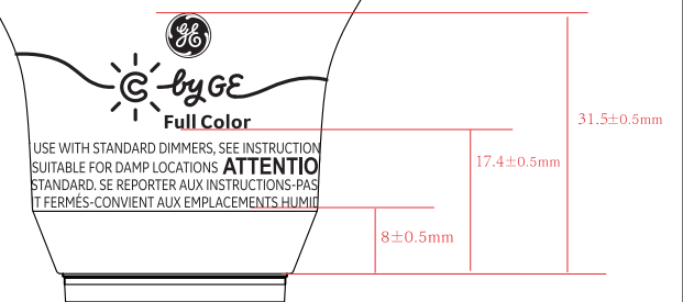
背面示意图
