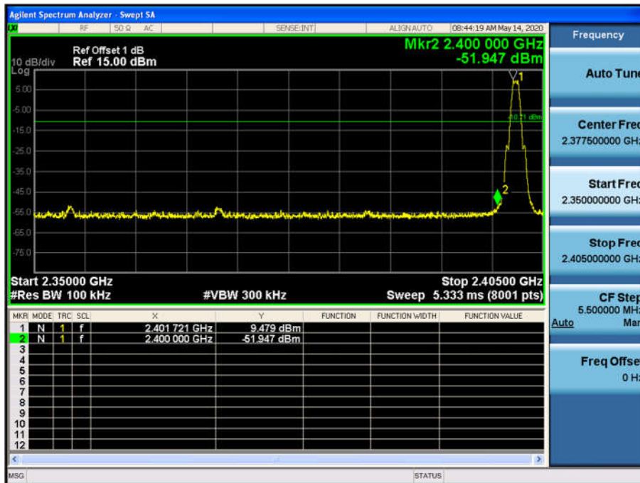
Mode 2 CH00(2402MHz)
