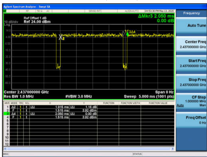
802.11n(20MHz)
