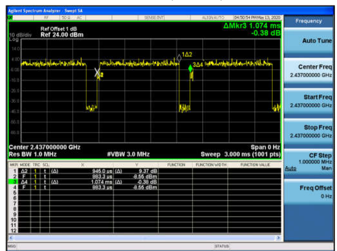
802.11n(40MHz)
