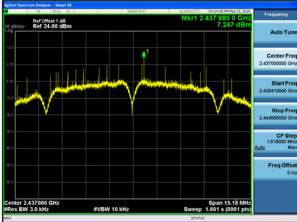
Mode 1 CH06(2437MHz)
