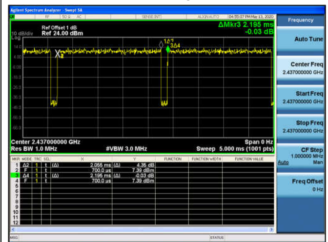
802.11n(40MHz)
