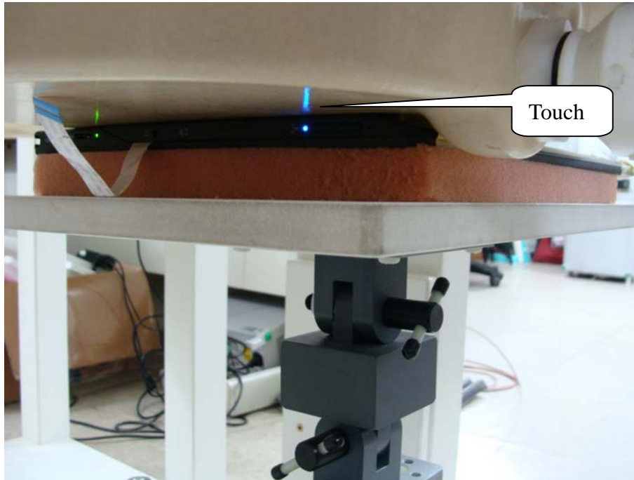
EUT Back (2.4G)
