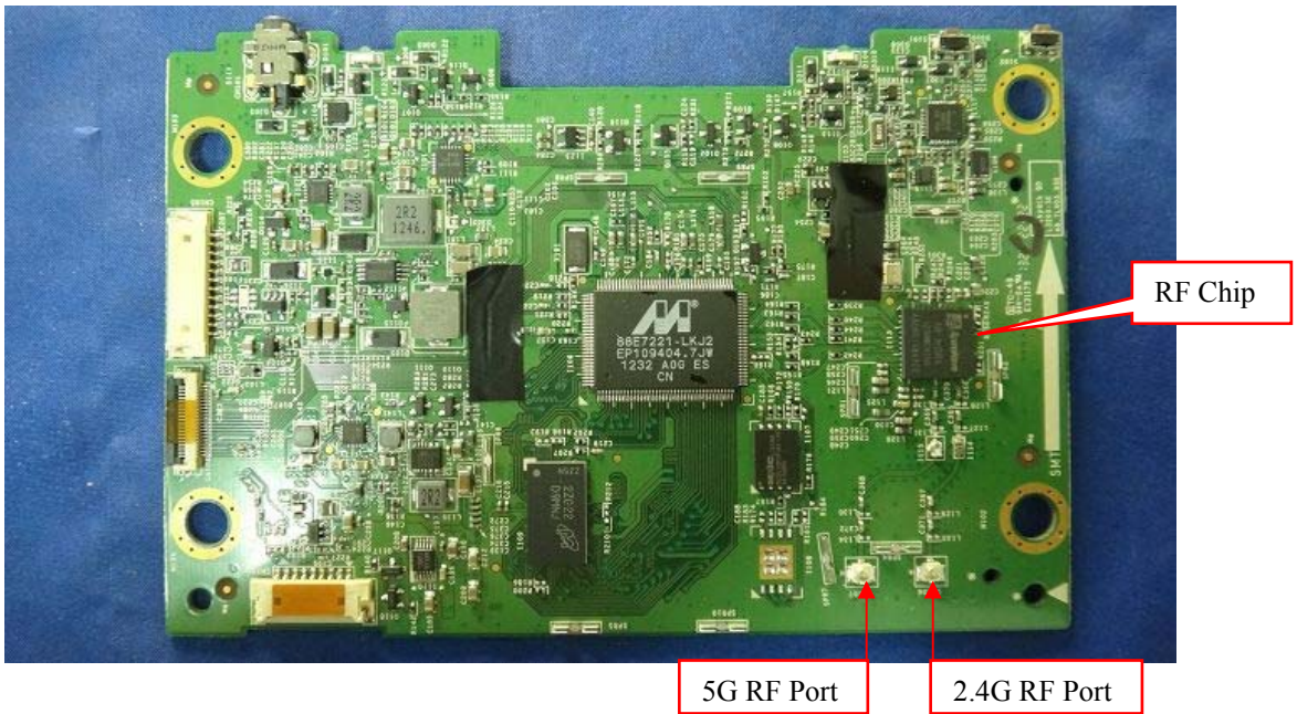
(13) EUT Photo
