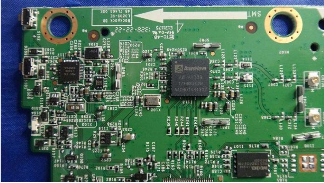
(14) EUT Photo
