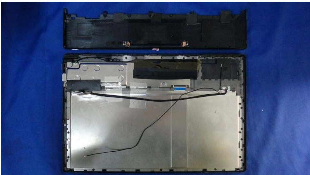
(21) EUT Photo
