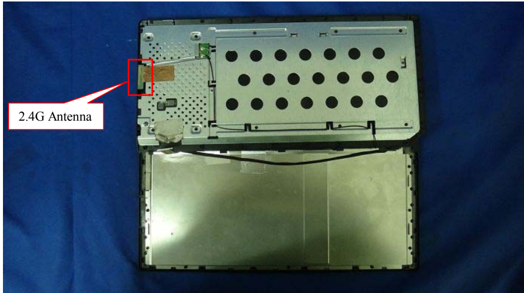
(8) EUT Photo
