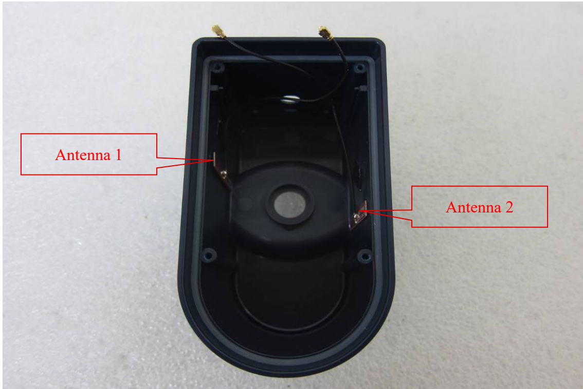
EUT 4 Antenna 1
