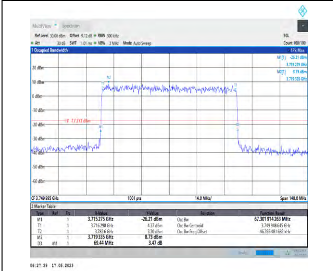
1-N78-3700-3800-PC1-30-70-M-9-CP-256QAM-Outer _Full-189@0-Ant1-67.302-69.440-≤70-PASS
