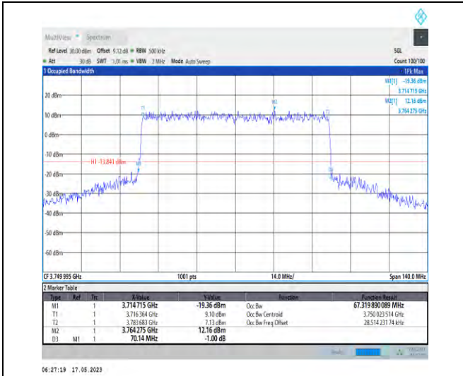
1-N78-3700-3800-PC1-30-70-M-7-CP-16QAM-Outer _Full-189@0-Ant1-67.32-70.140-≤70-PASS
