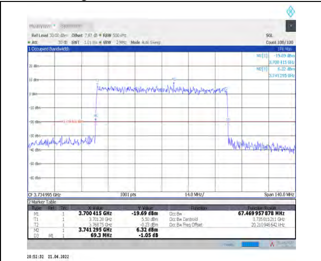
1-N78-3700-3800--30-70-L-9-CP-256QAM-Outer_Fu II-189@0-Ant1-67.47-69.300-≤70-PASS
