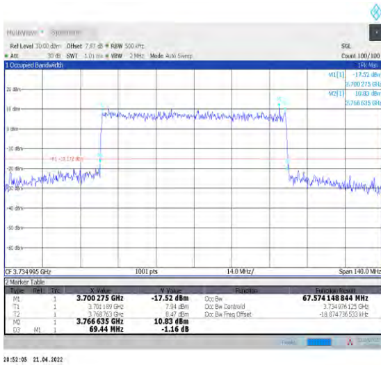
1-N78-3700-3800--30-70-L-6-CP-QPSK-Outer_Full-1 89@0-Ant1-67.574-69.440-≤70-PASS
