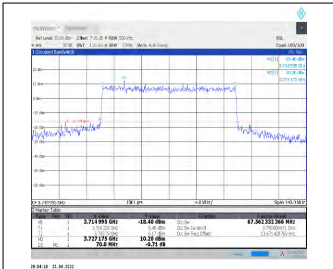
1-N78-3700-3800--30-70-M-7-CP-16QAM-Outer_Full -189@0-Ant1-67.562-70.000-≤70-PASS
