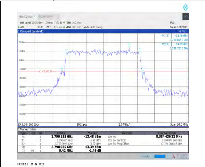
1-N78-3700-3800--30-10-H-4-DFT-64QAM-Outer_Fu II-24@0-Ant1-8.584-9.420-≤10-PASS
