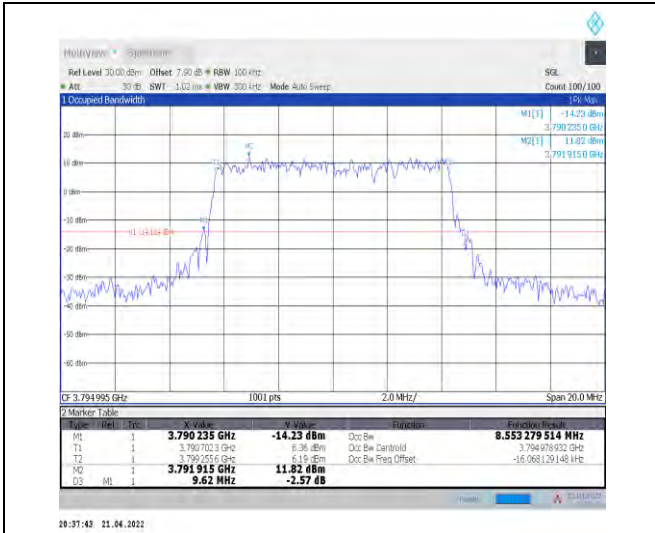
1-N78-3700-3800--30-10-H-3-DFT-16QAM-Outer_Fu II-24@0-Ant1-8.553-9.620-≤10-PASS
