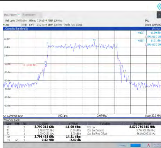
1-N78-3700-3800--30-10-M-9-CP-256QAM-Outer_Full -24@0-Ant1-8.582-9.420-≤10-PASS
