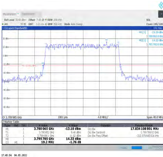
1-N78-3700-3800--30-20-H-3-DFT-16QAM-Outer_Fu II-50@0-Ant1-17.834-19.200-≤20-PASS
