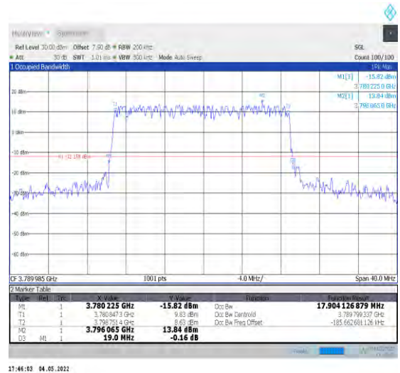
1-N78-3700-3800--30-20-H-4-DFT-64QAM-Outer_Fu II-50@0-Ant1-17.904-19.000-≤20-PASS
