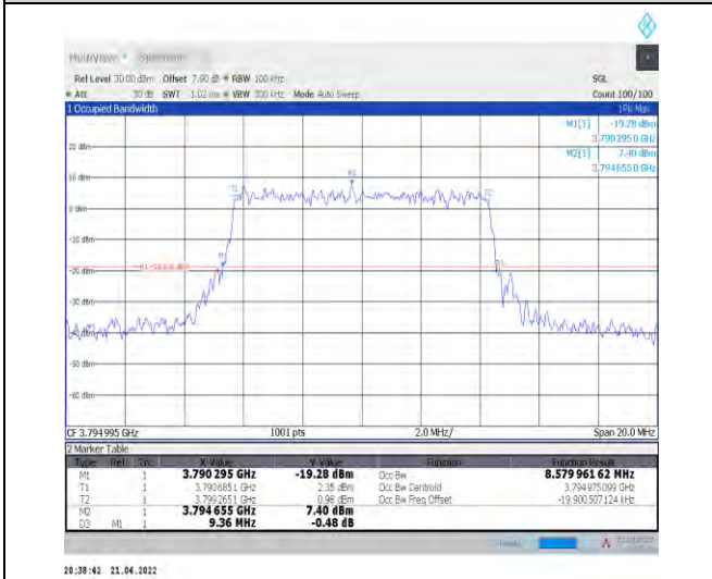
1-N78-3700-3800--30-10-H-9-CP-256QAM-Outer_Fu II-24@0-Ant1-8.58-9.360-≤10-PASS
