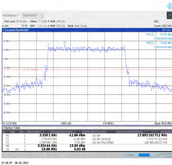
1-N78-3450-3550--30-20-H-3-DFT-16QAM-Outer_Fu II-50@0-Ant1-17.893-19.080-≤20-PASS
