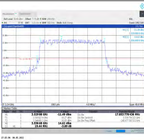
1-N78-3450-3550--30-20-H-1-DFT-QPSK-Outer_Full -50@0-Ant1-17.854-19.440-≤20-PASS
