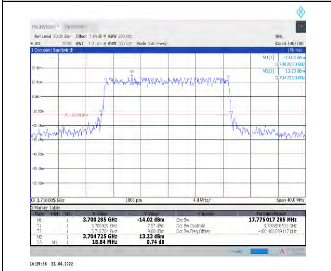
1-N77-3700-3980--30-20-L-1-DFT-QPSK-Outer_Full -50@0-Ant1-17.775-18.840-≤20-PASS
