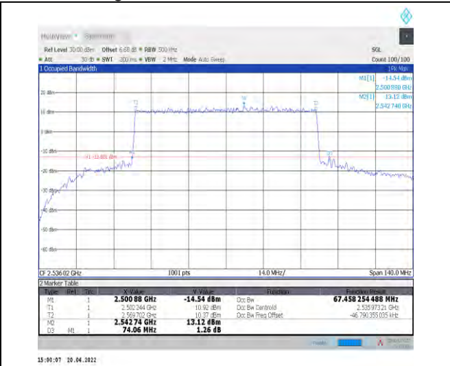
1-N41--30-70-L-7-CP-16QAM-Outer_Full-189@0-Ant1 -67.458-74.060-≤70-PASS
