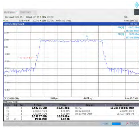
1-N41--30-20-M-9-CP-256QAM-Outer_Full-51@0-A nt1-18.251-19.960-≤20-PASS
