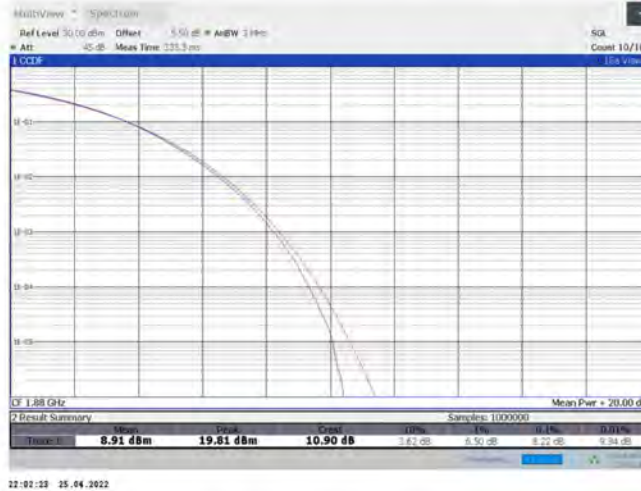
2-2-20MHz-20MHz-QPSK-QPSK-18801-18999-100RB#0-100RB#0
