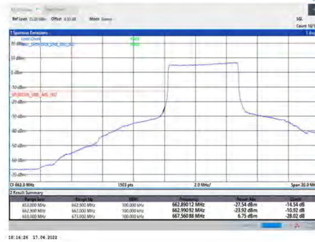
Band71-5MHz-QPSK-133147-25RB#0
