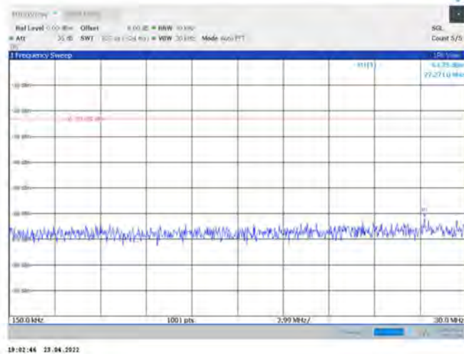
Band42-20MHz-QPSK-42190-1RB#0-Range2:0.15~30MHz
