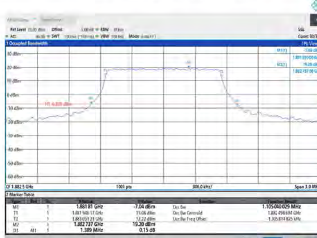
Band25-1.4MHz-QPSK-26365-6RB#0
