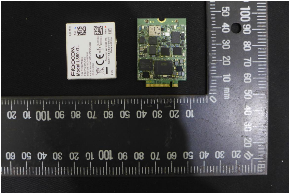
Module: L850-GL
