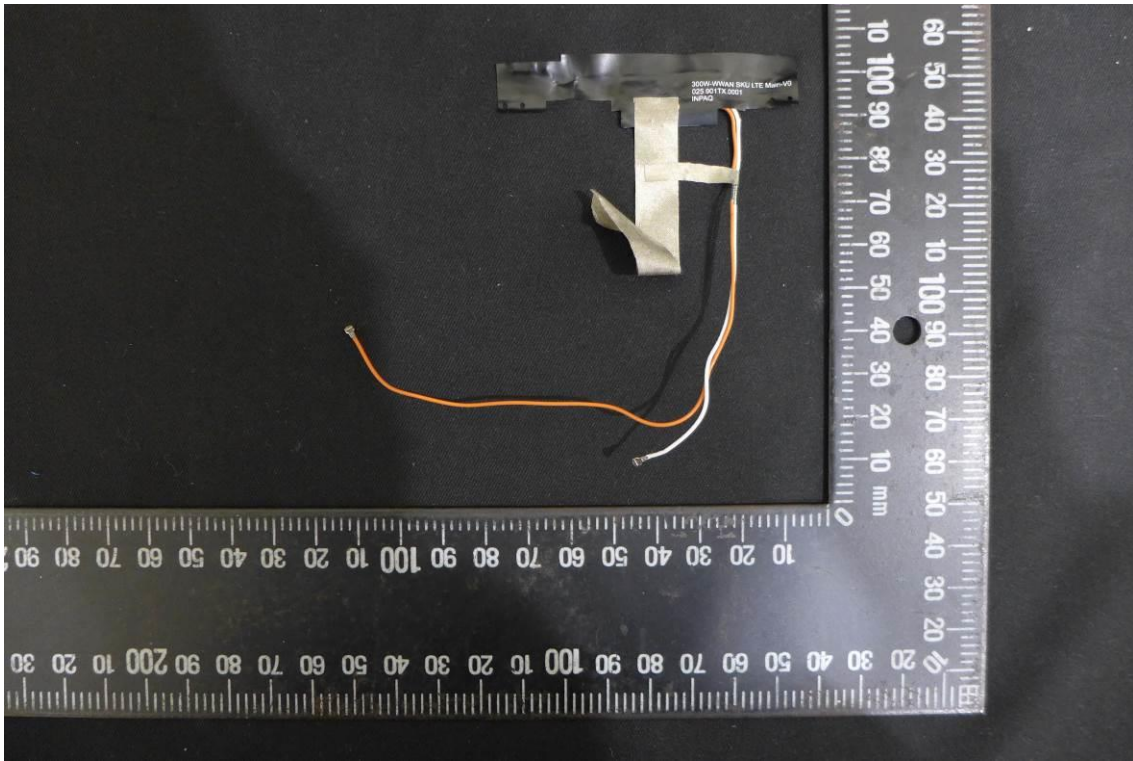
Antenna: INPAQ/025.901TX.0001
